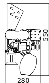
Szarufa rögzítés
