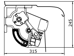
Homlokzati rögzítés védőtetővel
