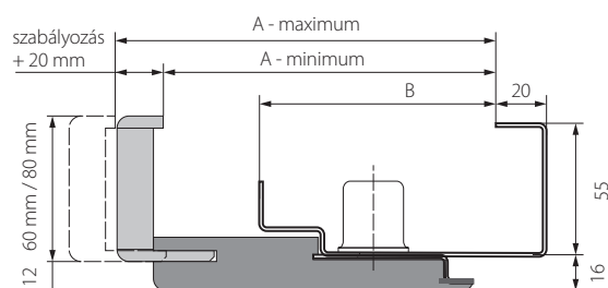
PROJECT Prémium tok keresztmetszete
