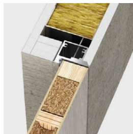
Falc nélküli (kifelé nyíló) - jobbos ajtó
